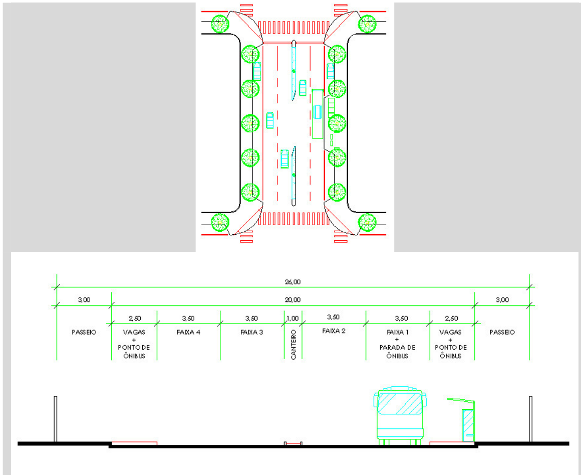
FIGURA 04 VIA EIXO/ARTERIAL - MÃO ÚNICA
