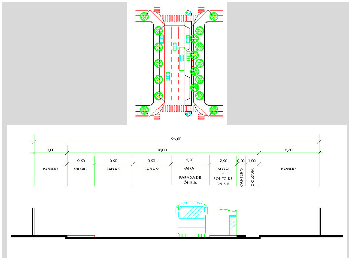
FIGURA 04 VIA EIXO/ARTERIAL - MÃO ÚNICA - CICLOVIA
