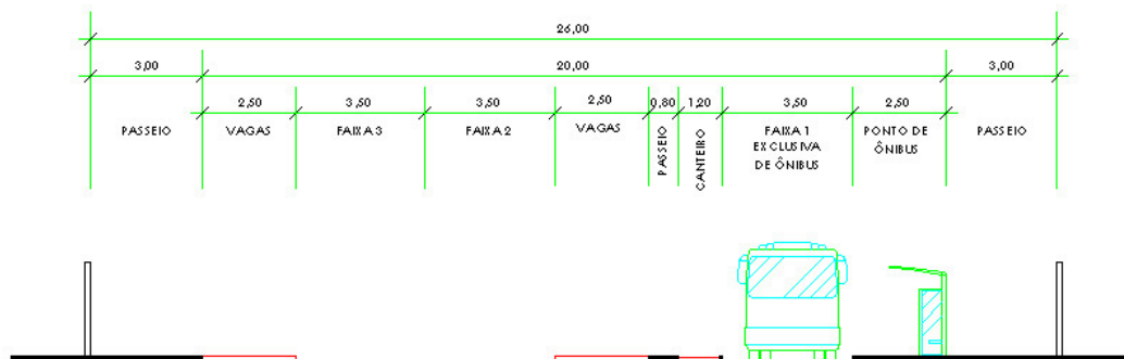
FIGURA 04 VIA EIXO/ARTERIAL - MÃO ÚNICA - ÔNIBUS
