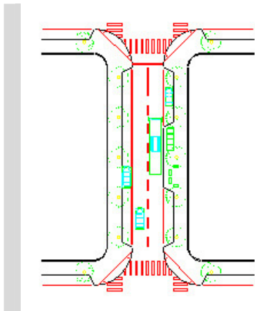
FIGURA 03 VIA COLETORA - MÃO ÚNICA
