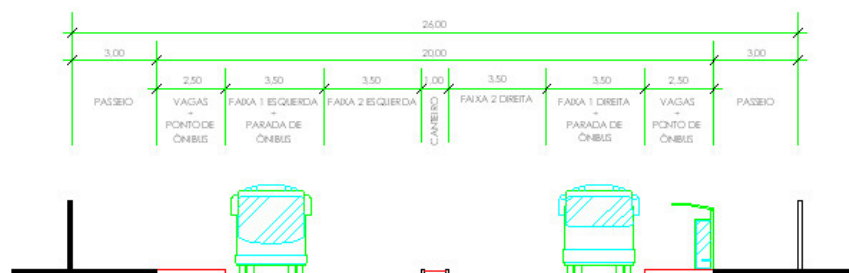
FIGURA 04 VIA EIXO/ARTERIAL - MÃO DUPLA
