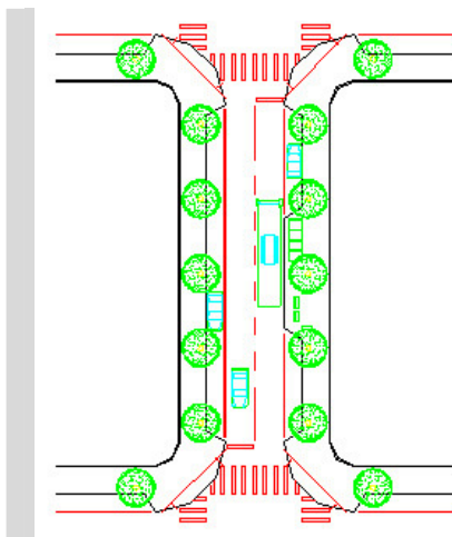
FIGURA 04 VIA COLETORA - MÃO DUPLA
